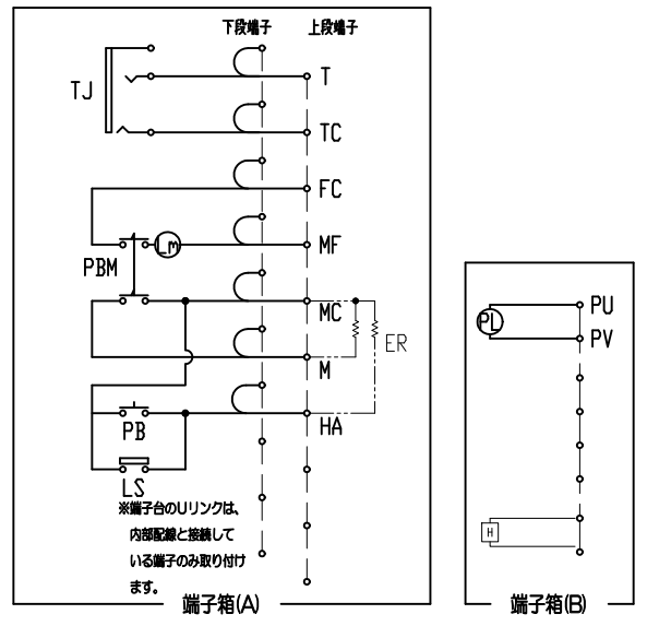
結線図
